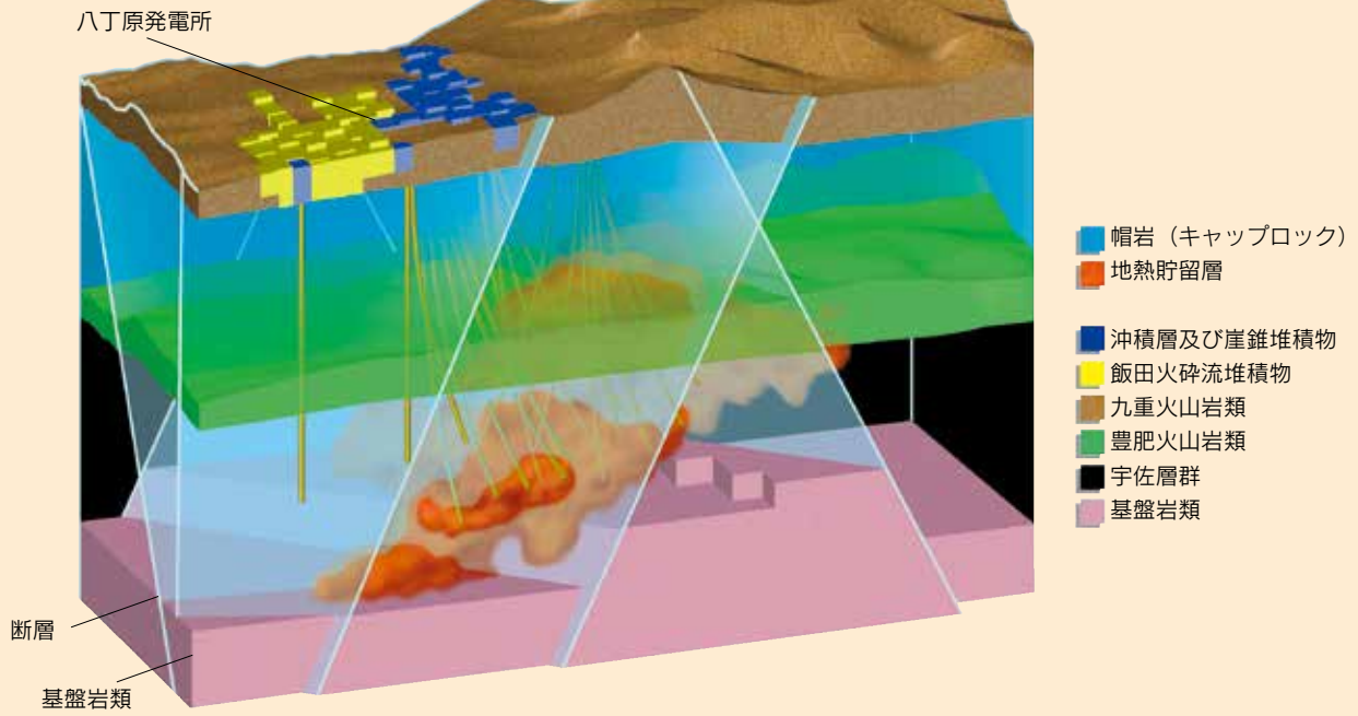
3次元コンピュータ・グラフィックによる地熱構造図（断面図）
