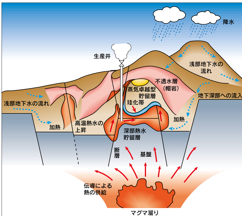
■地熱構造概念図
